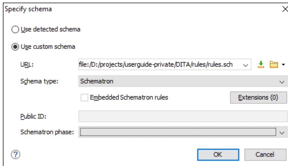
Figure 241. Specify Schema Dialog Box
